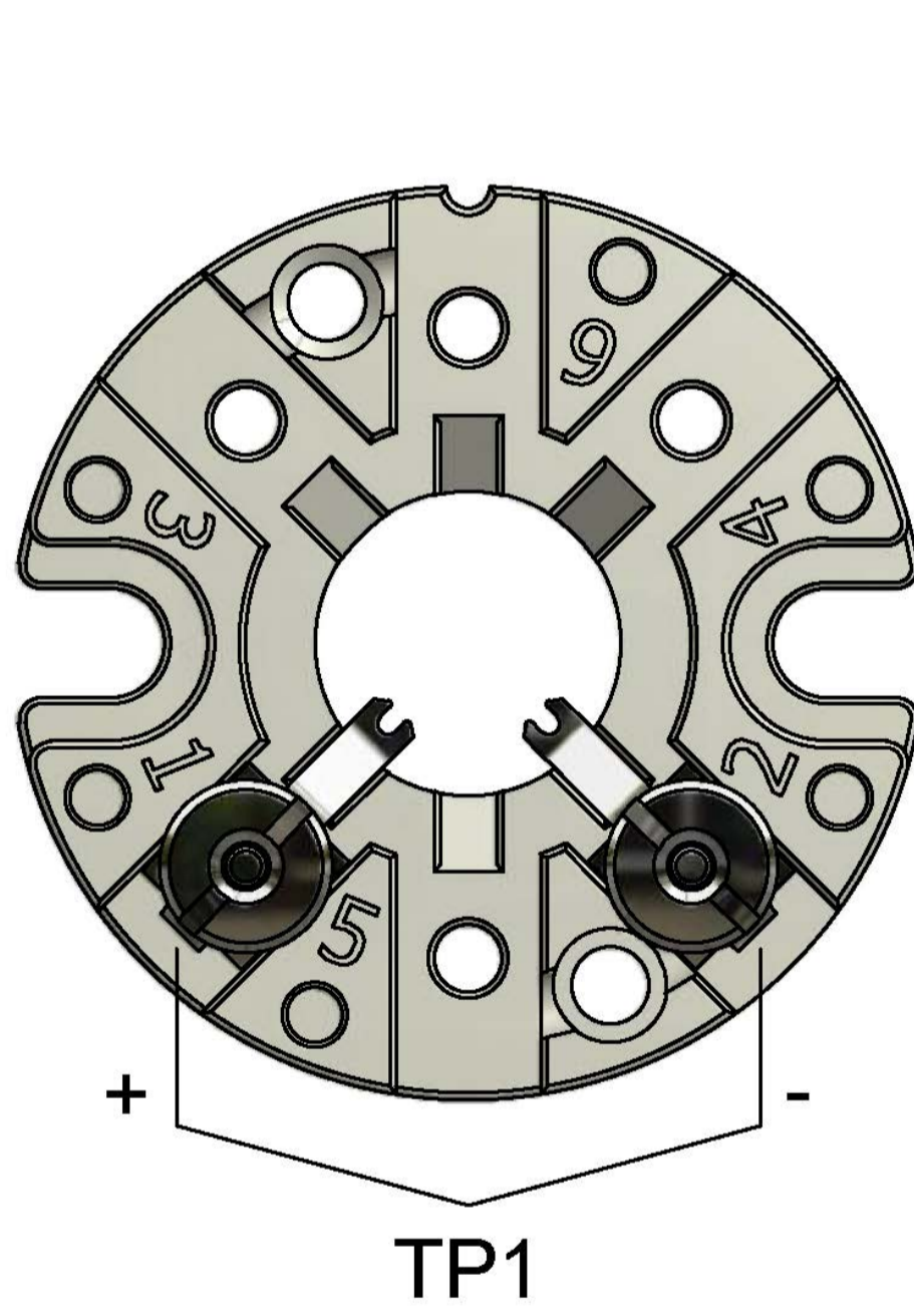
Anschlusssocket 1 Thermopaar
